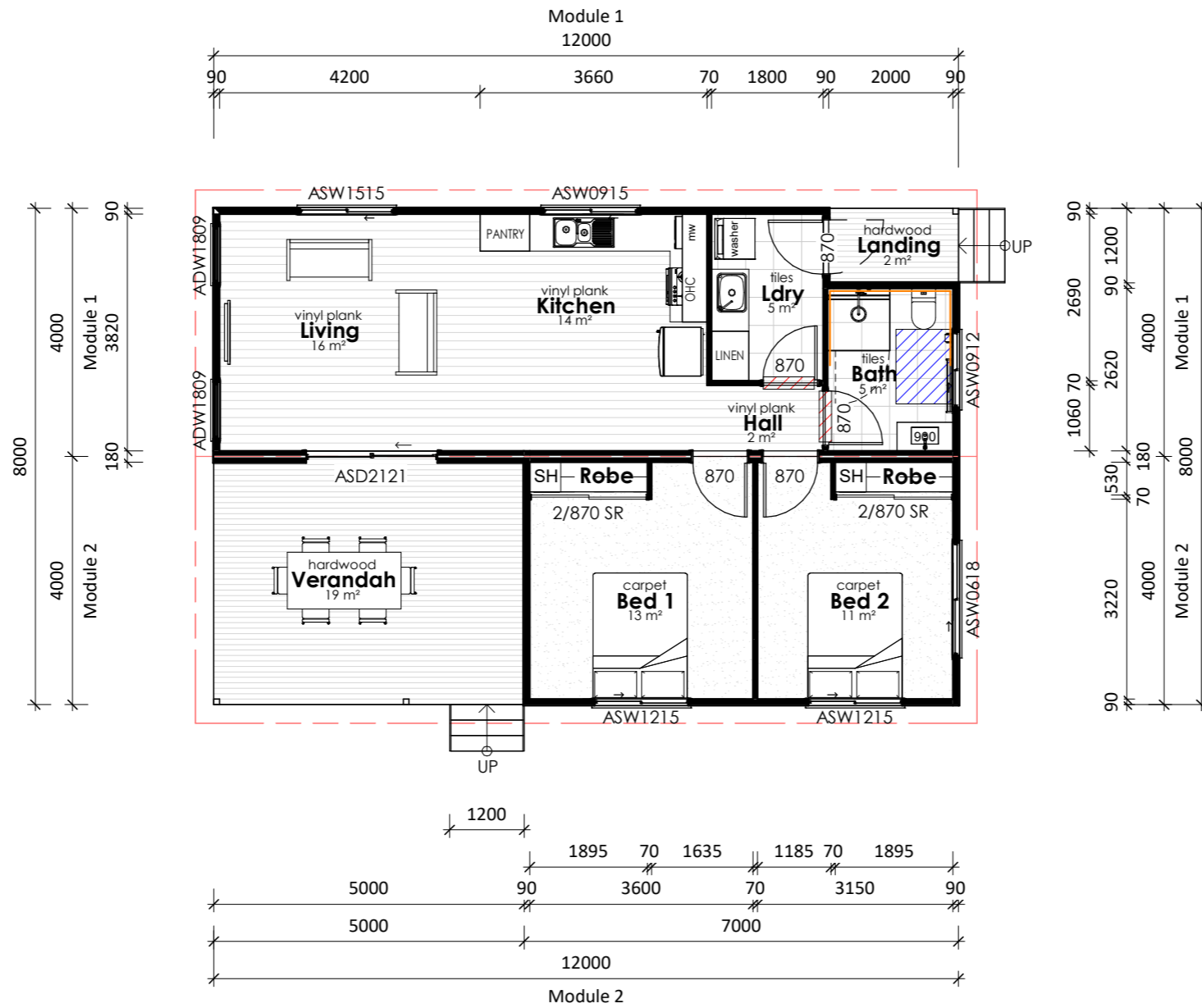
Plan Floor Plan 1 : 100
