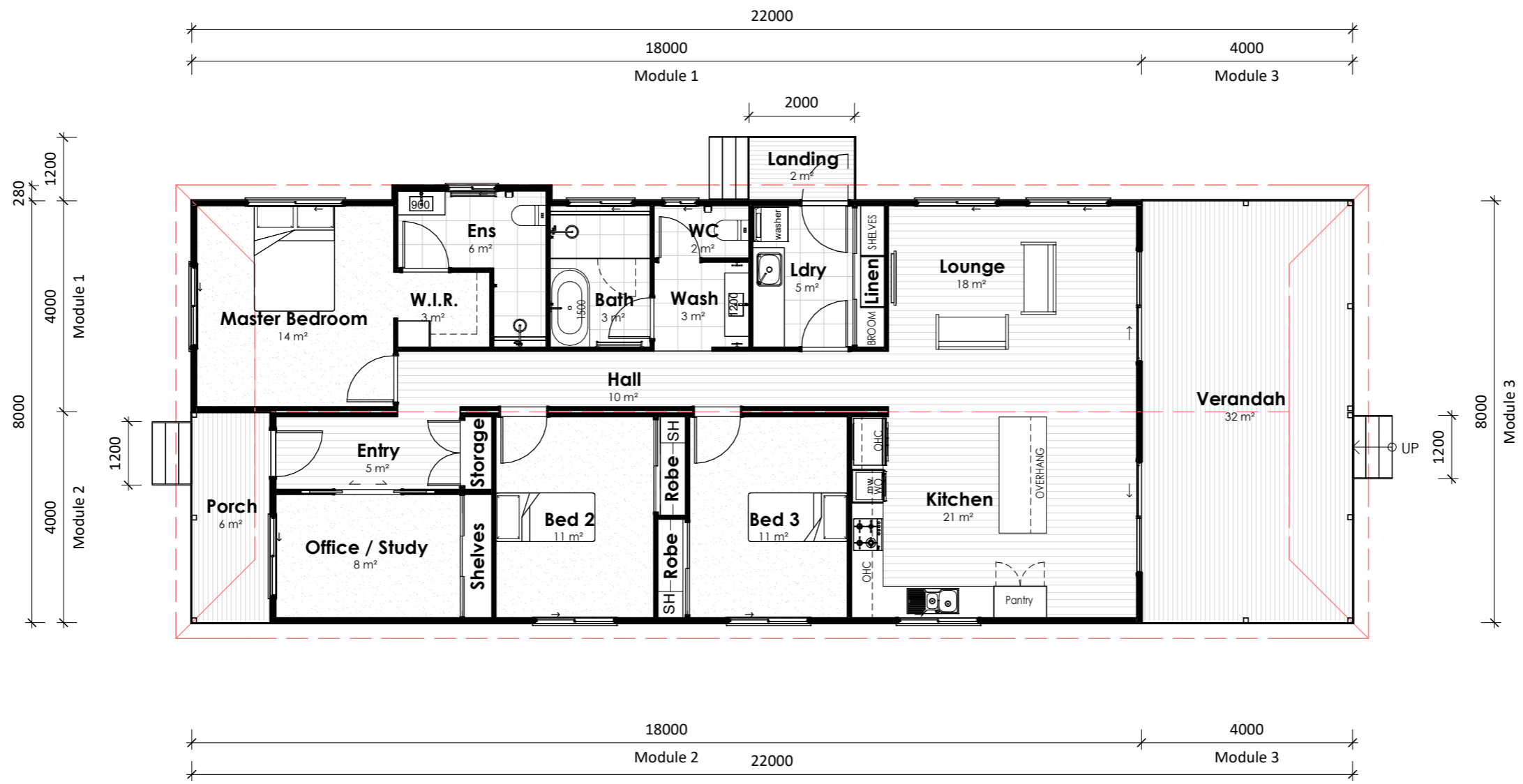
Plan Floor Plan 1 : 100
