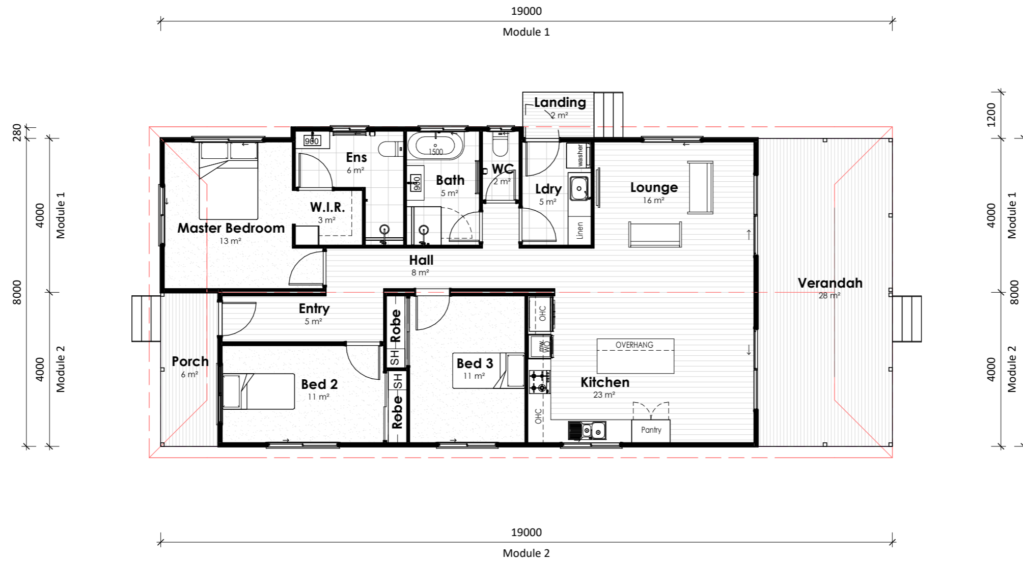
Plan Floor Plan 1 : 100
