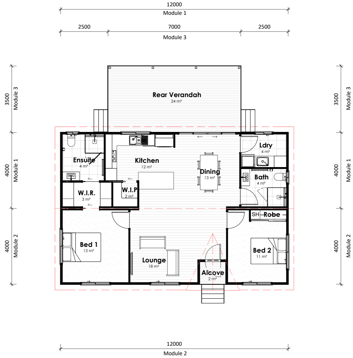
Plan Floor Plan 1 : 100
