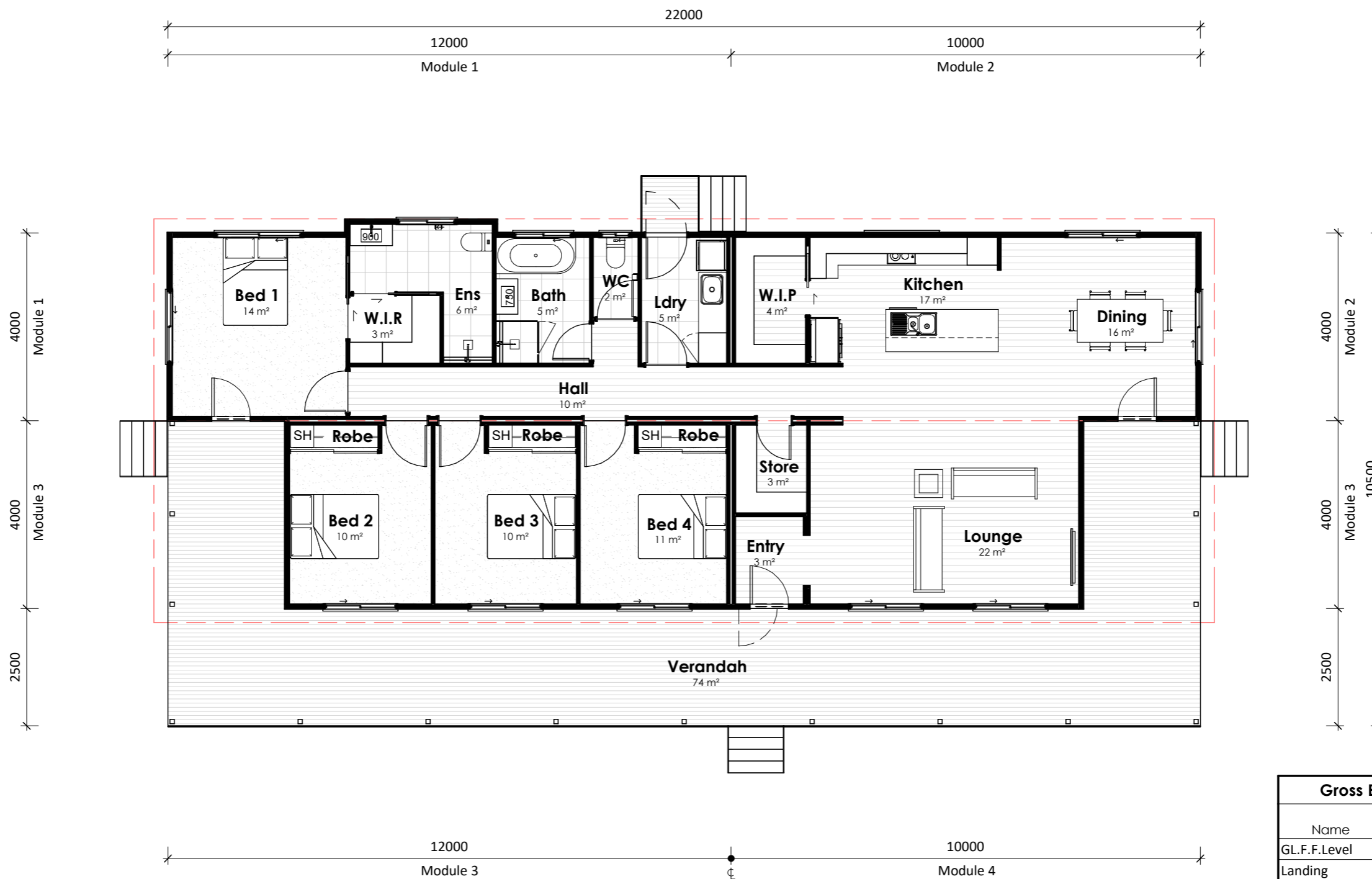
Plan Floor Plan 1 : 100
