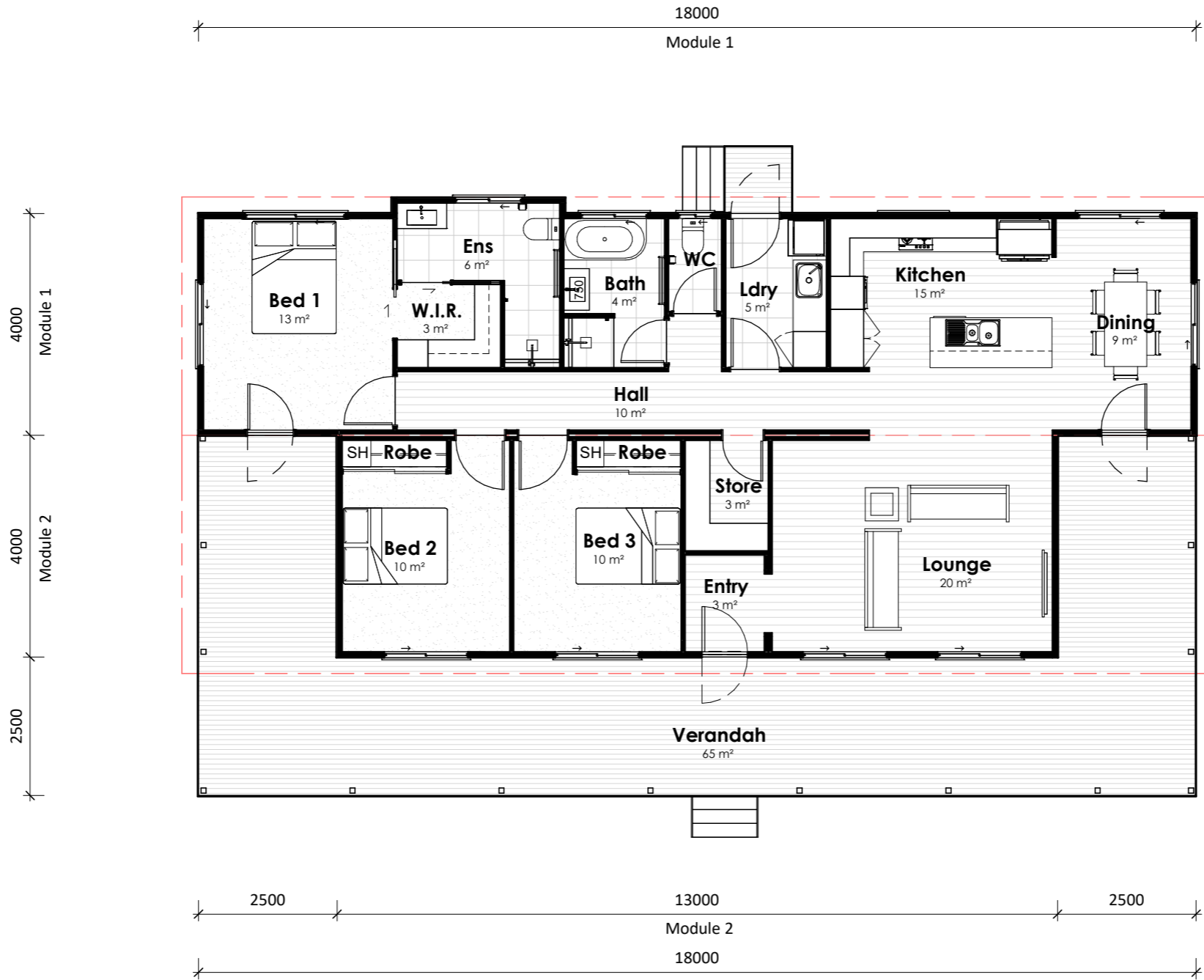
Plan Floor Plan 1 : 100
