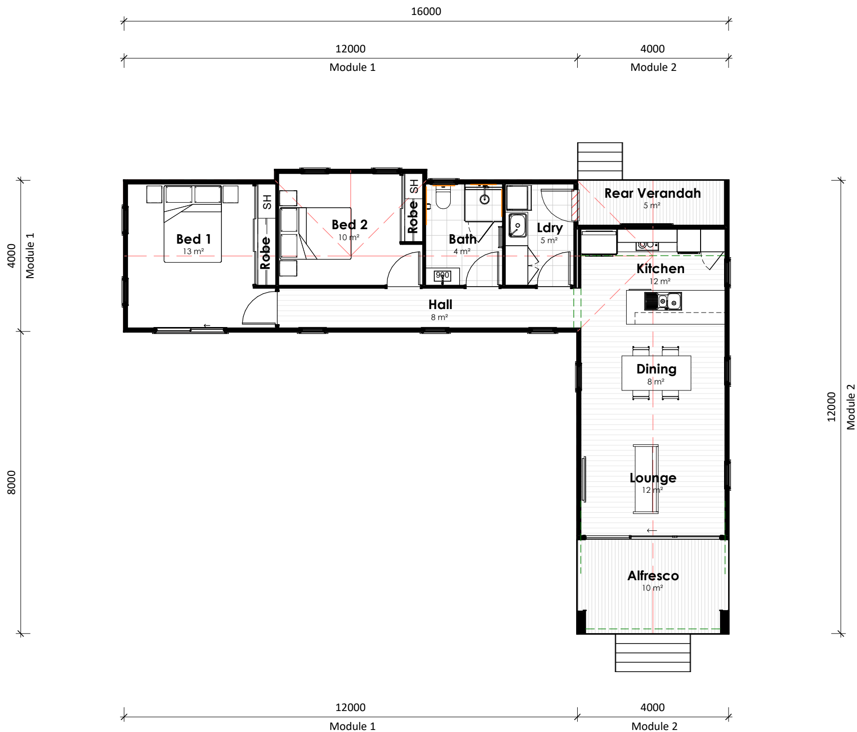
Plan Floor Plan 1 : 100
