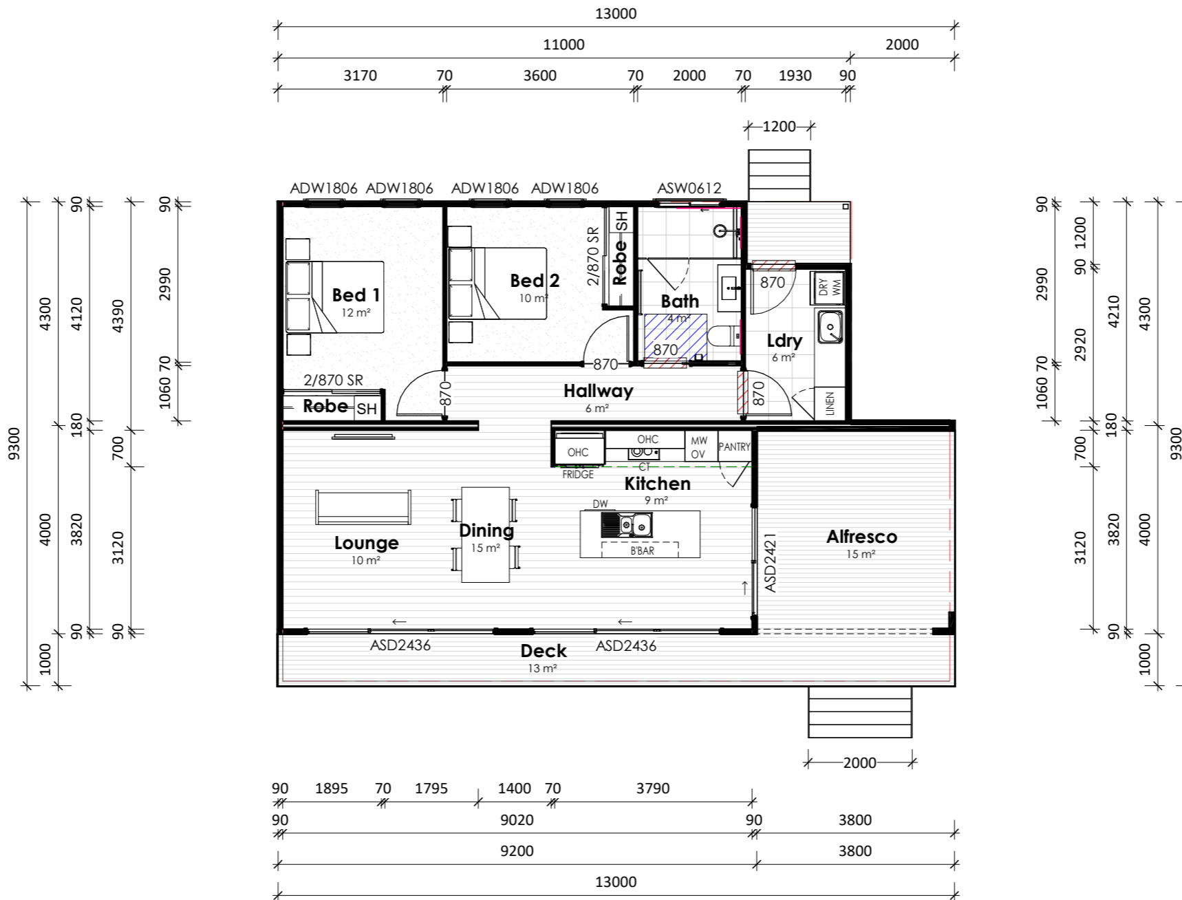
Plan Floor Plan 1 : 100
