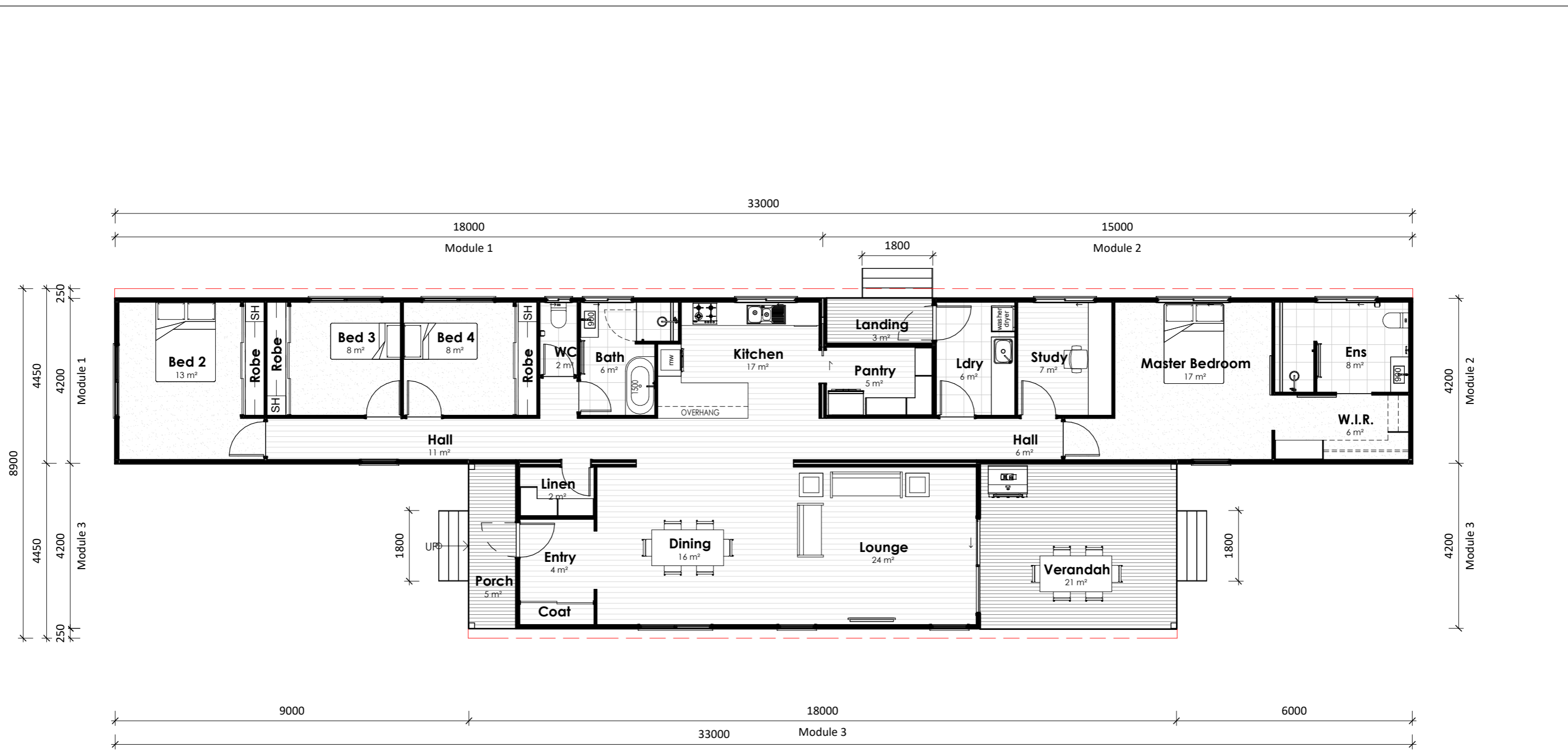
Plan Floor Plan 1 : 100
