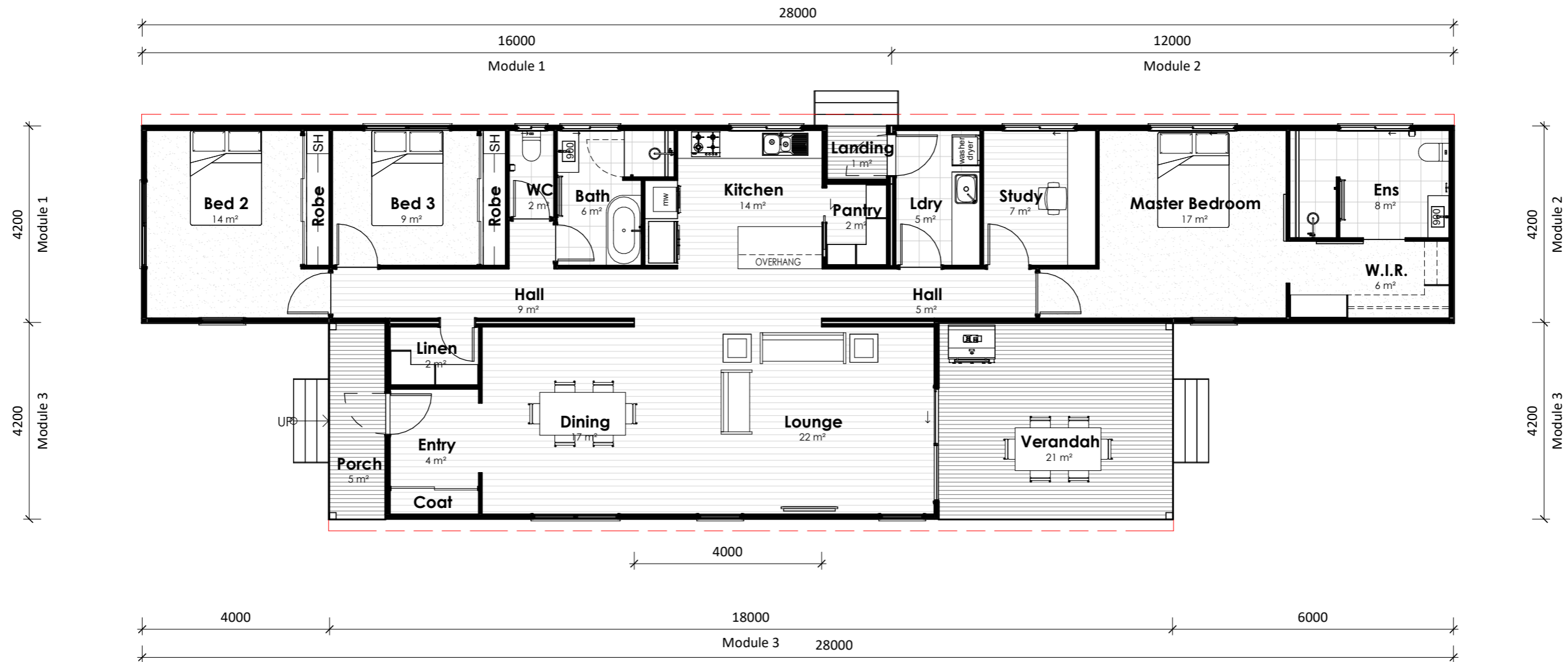
Plan Floor Plan 1 : 100
